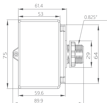
螺栓安装 UM08
