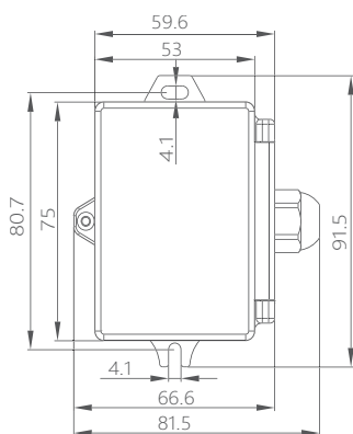
平面安装 UM09
